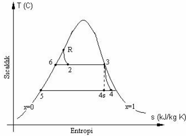
Şekil 3. Tek flaşlı santralde jeoakışkanın sıcaklık-entropi diyagramı
