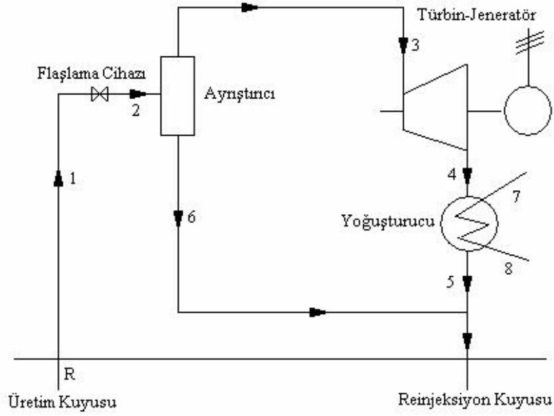
Şekil 2. Tek flaşlı jeotermal güç santralinin tesis şeması
