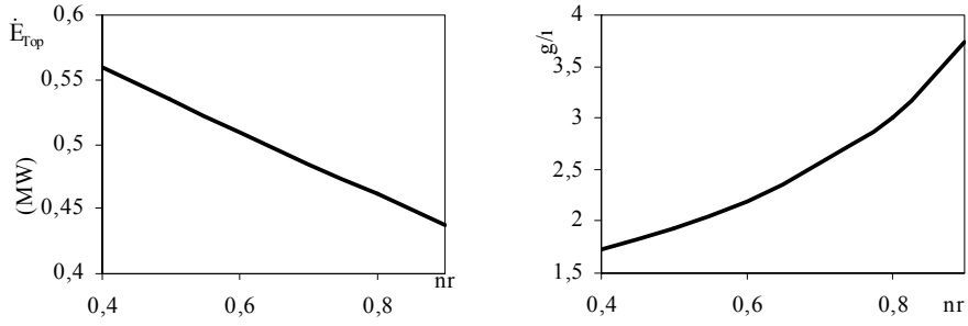
Şekil 4. a) Rejeneratör verimi ile toplam ekserji değışimi b) Rejeneratör verimi ile güç/ısı oranı değışimi
