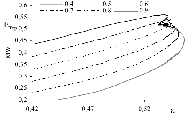
Şekil 5. Çeşitli rejeneratör verimleri için ekserji verimi ile toplam ekserji değışimi
