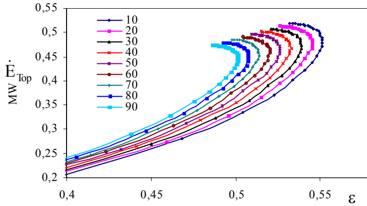
Şekil 12. Çeşitli DTp değerleri için ekserji verimi ile toplam ekserji değişimi
